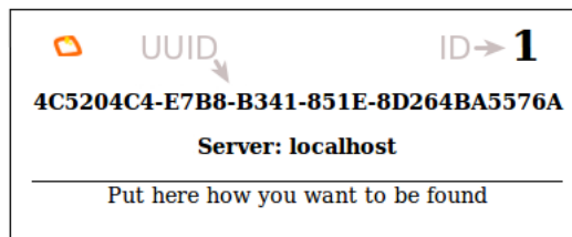
Figura 2: Comando migasfree-label .
